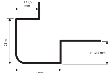
PEBDAC/ACS 125 échelle 1:1
