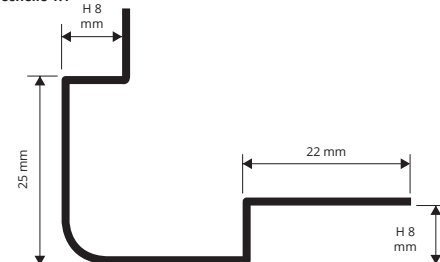
PEBDAC/ACS 08 échelle 1:1
