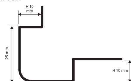
PEBDAC/ACS 10 échelle 1:1
